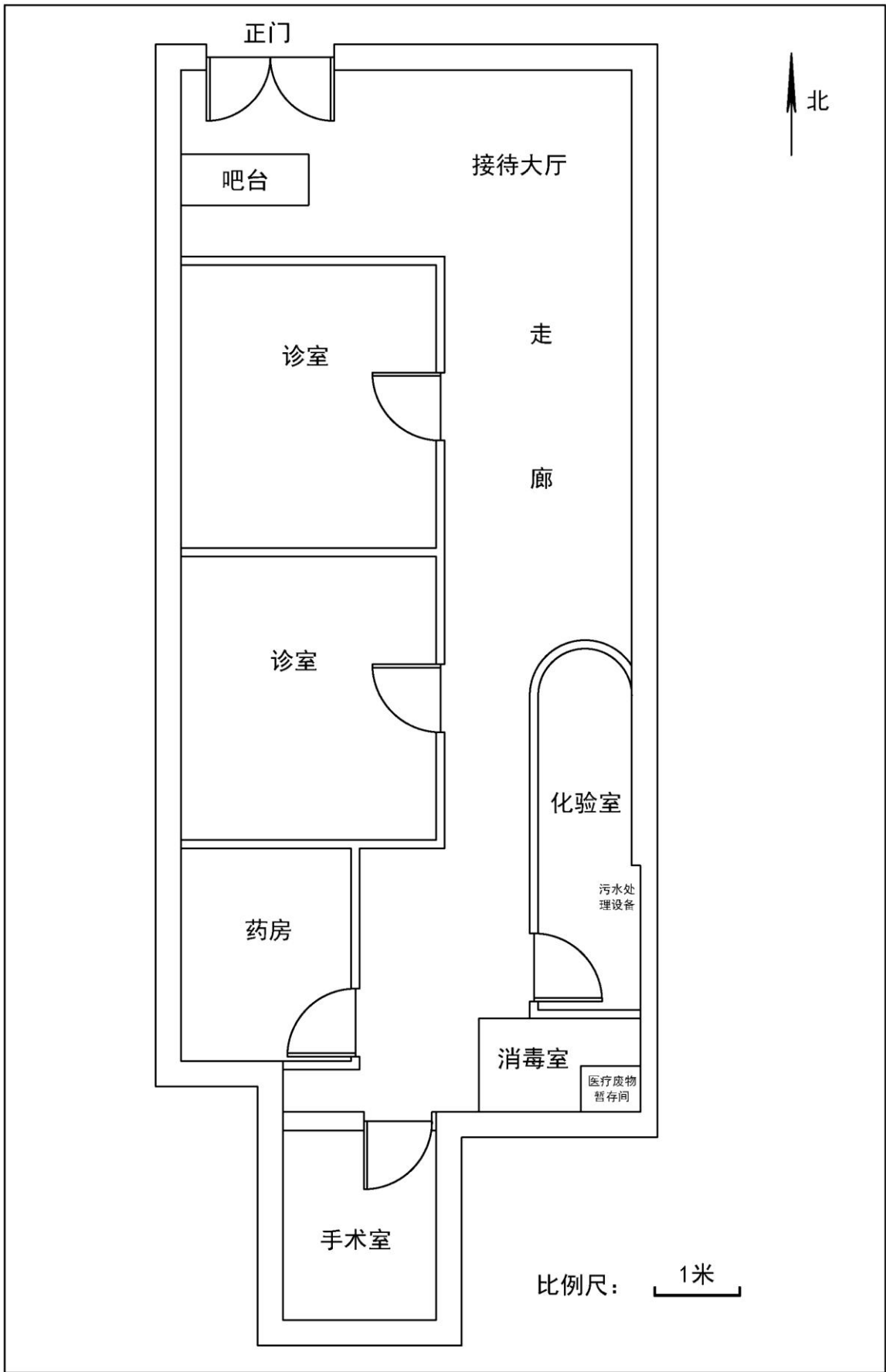
附图 3 建设项目平面布置图
