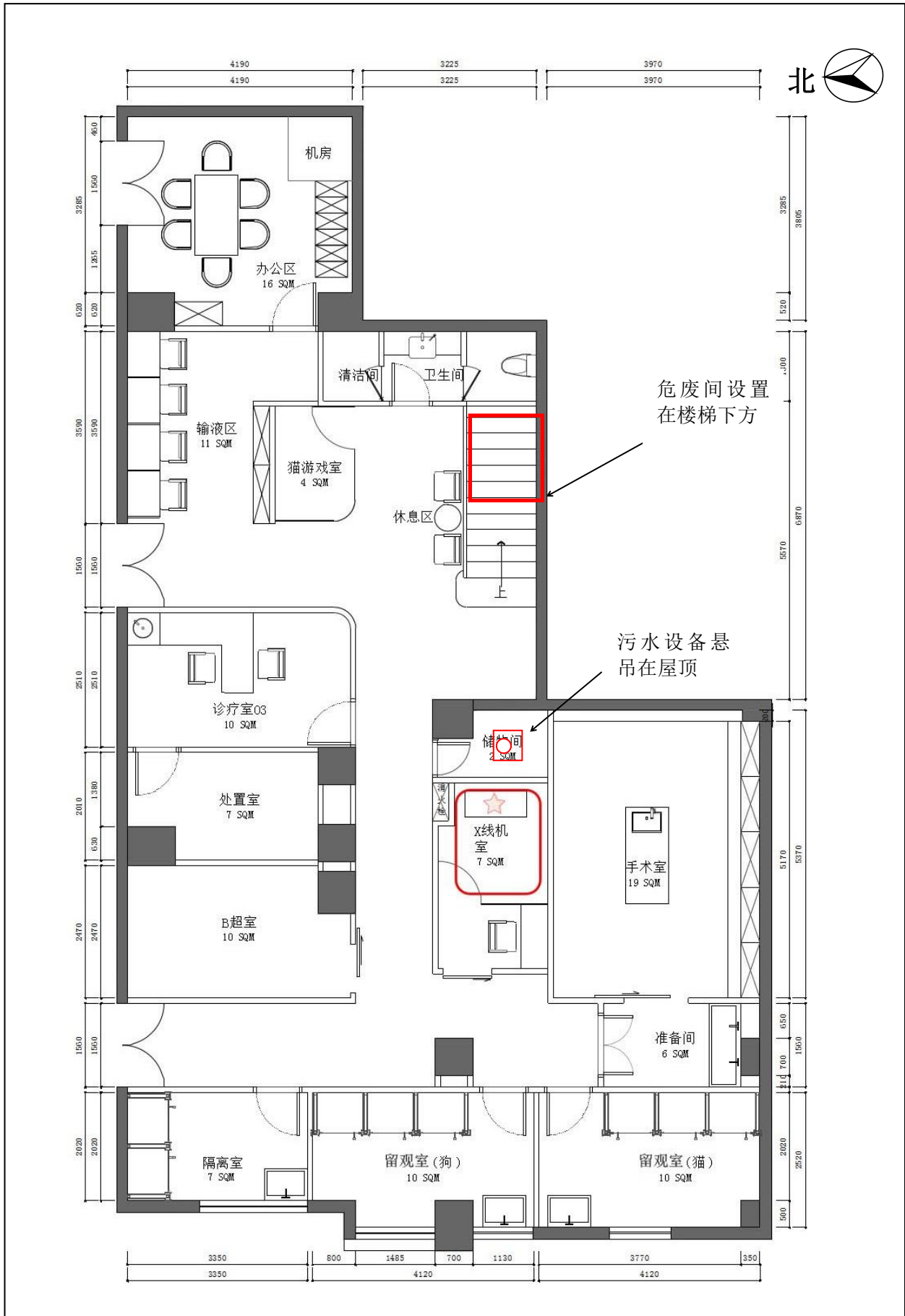
附图 3 建设项目地下一层平面布置图
