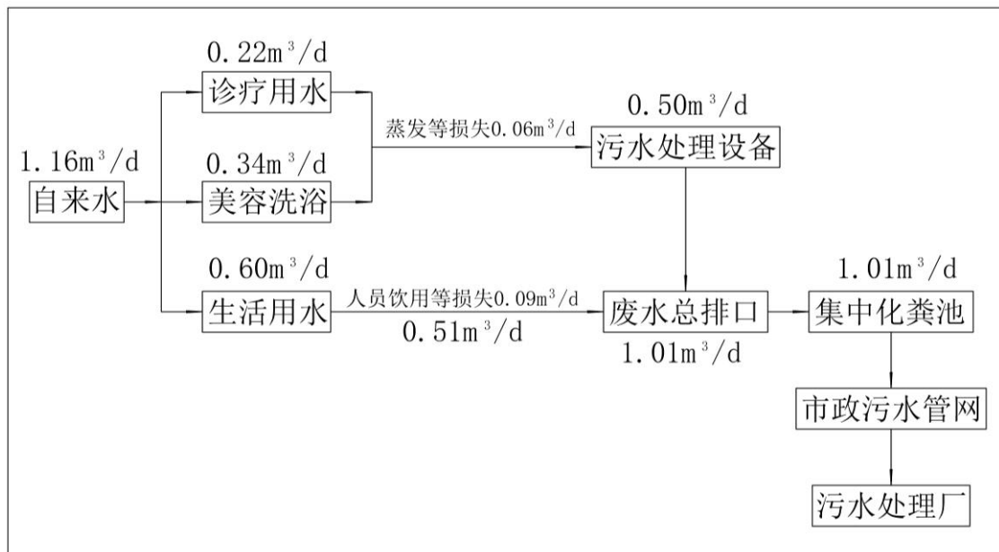
图 4 项目水平衡图
